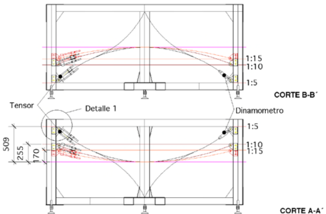
Figura 4 Marco de soporte.
